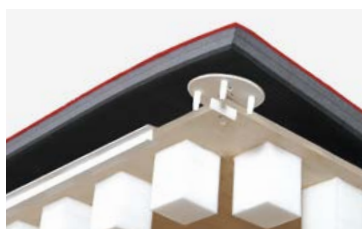
Detail van de plankenvloer en de rolmaten
